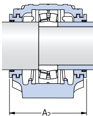
Obtunicaciones de laberinto Diseño S
