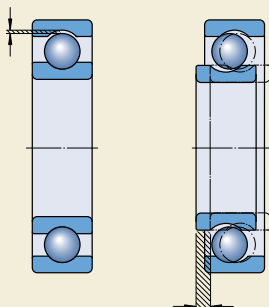
Juego axial interno
