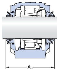
Obturaciones Taconite Diseño ND
