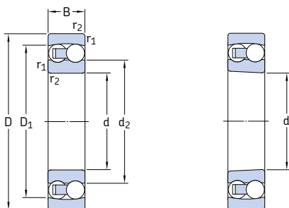
Agujero cil ndrico
