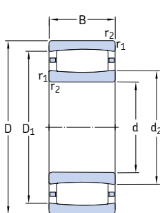
Agujero cilíndrico
