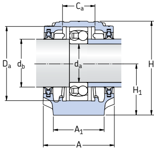
Obturaciones de doble labio Diseño G
