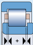
Juego axial interno de los rodamientos de rodillos cilíndricos de diseño NUP
