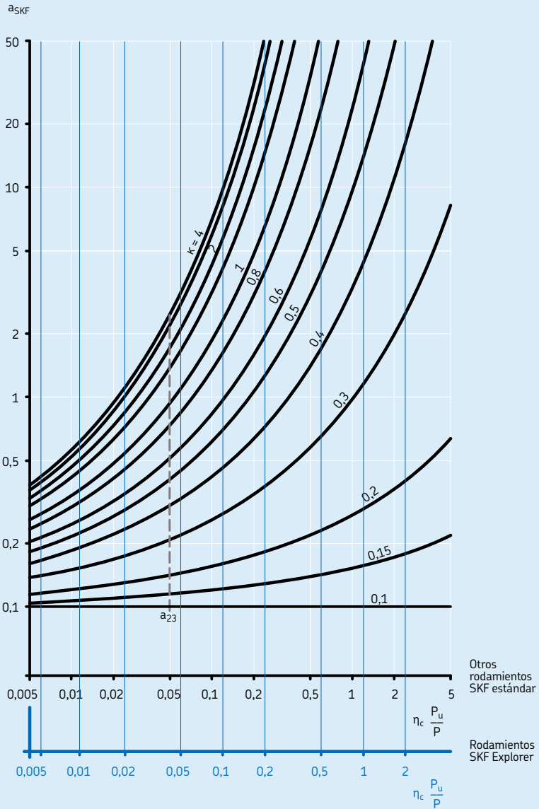
Factor a_{SKF} para rodamientos radiales de bolas
