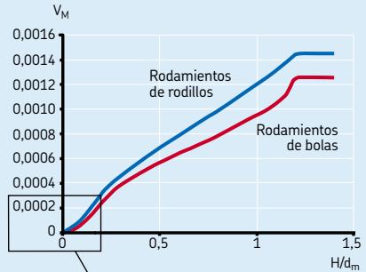
Variable de pérdida de energía por agitación del aceite V_M
