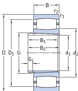
Rodamiento sobre un manguito de desmontaje de diseño AH
