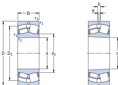
Agujero cil ndrico
