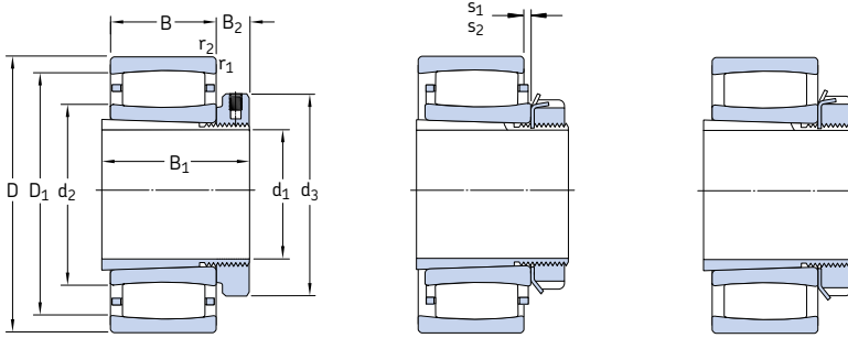
Rodamiento completamente lleno de rodillos sobre un manguito de fijación estándar
