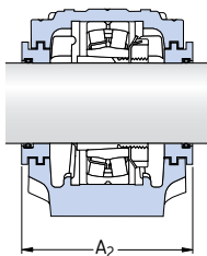
Obturaciones de laberinto Diseño S
