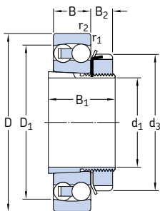
Rodamiento abierto
