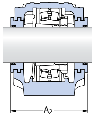
Obturaciones de laberinto Diseño S
