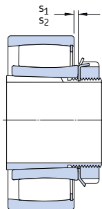
Rodamiento completamente lleno de rodillos sobre un manguito de fijación estándar
