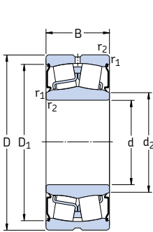
Agujero cilíndrico
