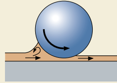
Flujo inverso del lubricante
