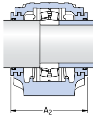
Obturaciones de laberinto Diseño S
