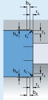
Acuerdos con chaflanes
