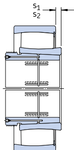
Rodamiento sobre un manguito de desmontaje de diseño AOH para el método de inyección de aceite
