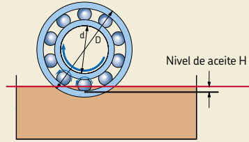
Nivel de aceite en un baño de aceite
