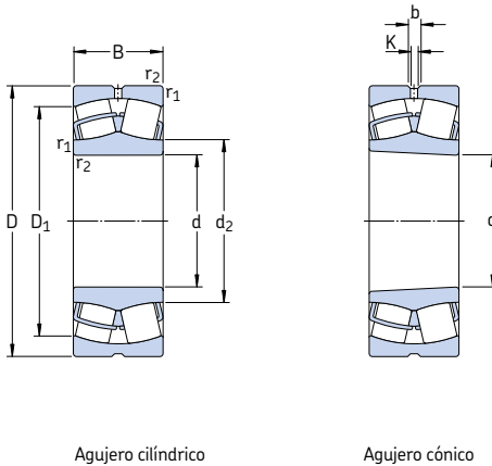
Agujero cilíndrico
