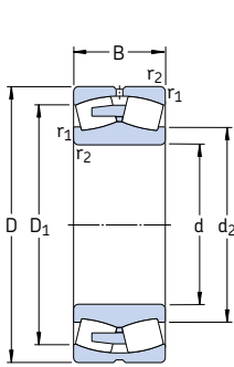
Agujero cil ndrico
