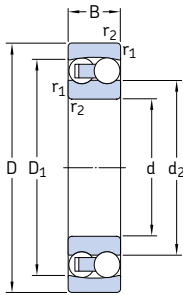
Agujero cil ndrico
