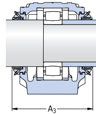
Obturaciones Taconite Diseño ND
