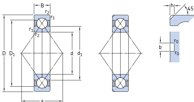
Rodamientos con un diseño básico
