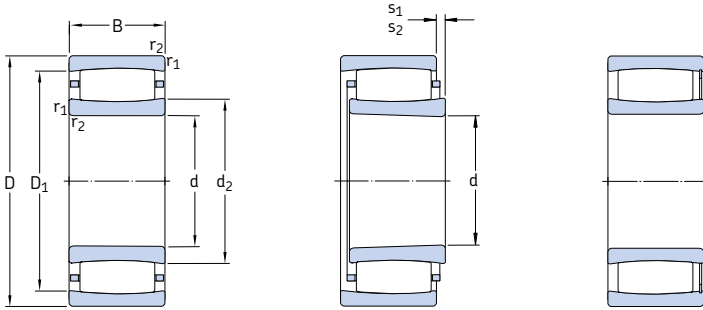
Agujero cilíndrico
