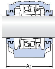
Obturaciones de laberinto Diseño S
