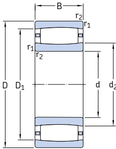
Agujero cilíndrico
